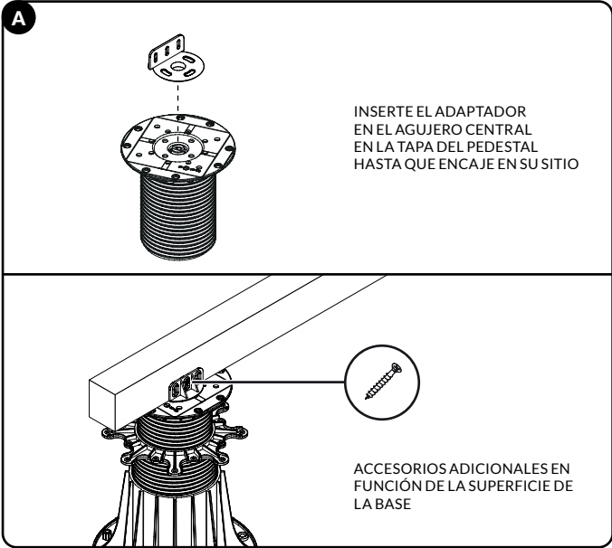
CABEZA DEL SOPORTE CON TORNILLO
